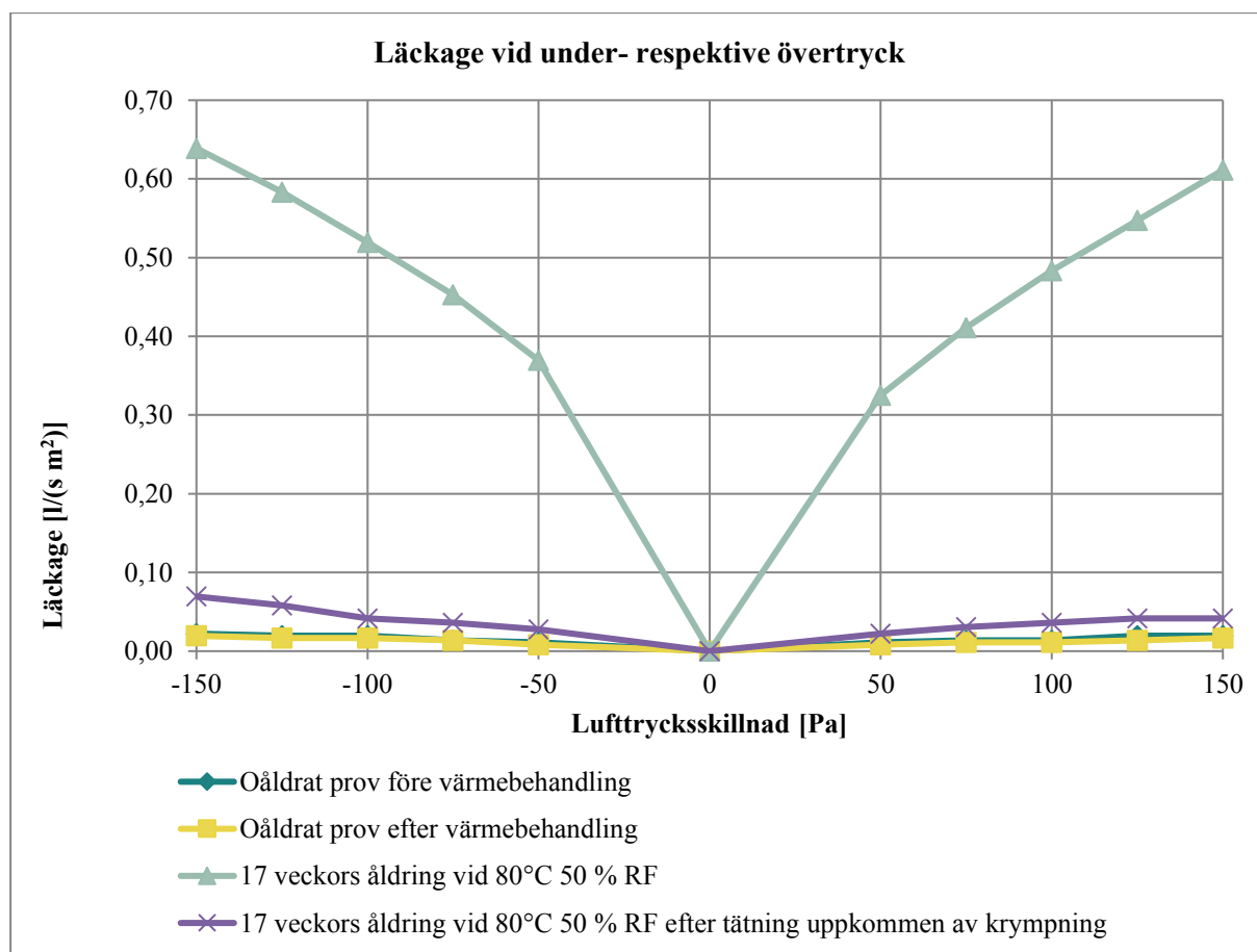
Diagram 13. Resultat från långtidsåldring av in-situ tillverkad provvägg med polyuretanisolerings.
