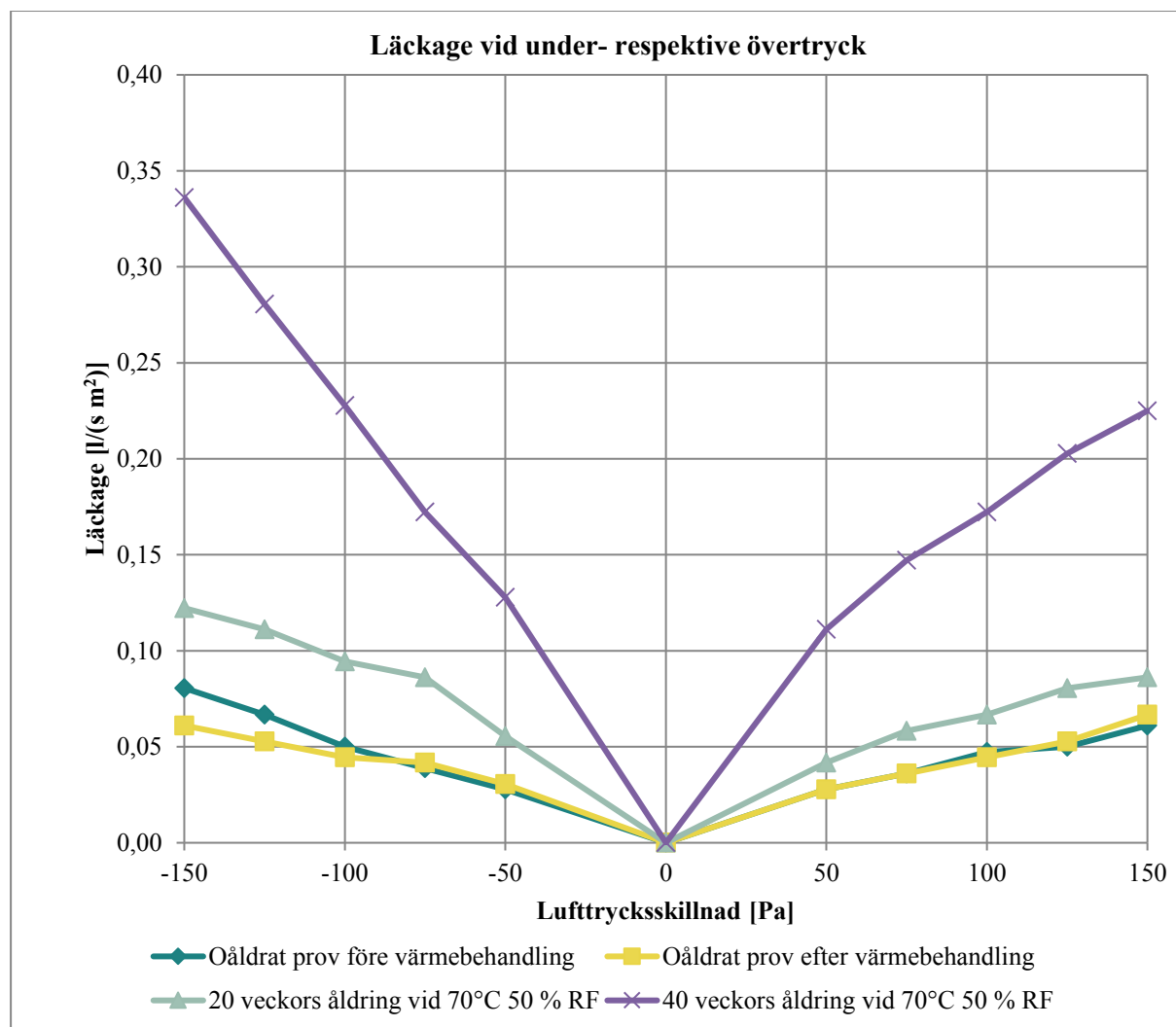
Diagram 7. Sammanställning av mätningar av luftläckaget då montage av lufttätthetssystemet har gjorts under ideala förhållanden och därefter långtidsåldring under 40 veckor vid 70°C 50 % RF.
