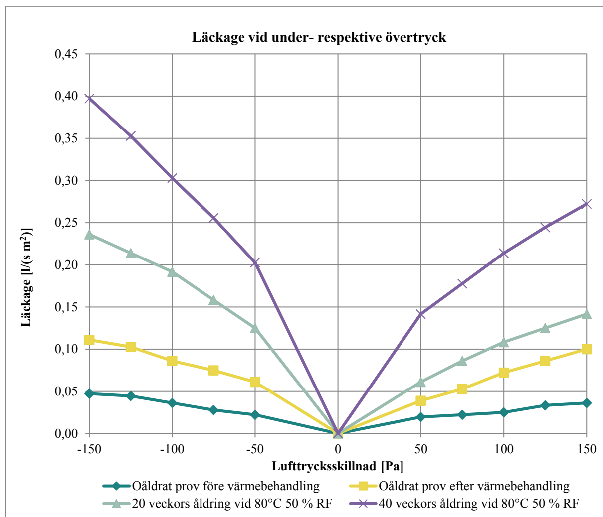
Diagram 9. Sammanställning av mätningar av luftläckaget då montaget av lufttätthetssystemet har gjorts under ideala förhållanden och därefter långtidsåldring under 40 veckor vid 80°C 50 % RF.
