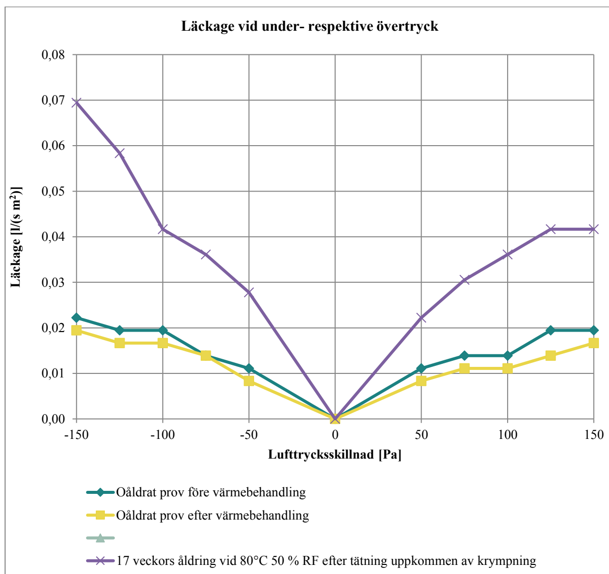
Diagram 14. Resultat från långtidsåldring av in-situ tillverkad provvägg med polyuretanisolering där läckage från krypning mellan stålram och väggkonstruktionen har tagits bort. Detta är alltså samma konstruktion som redovisas i diagram 8 men där information har tagits bort.
