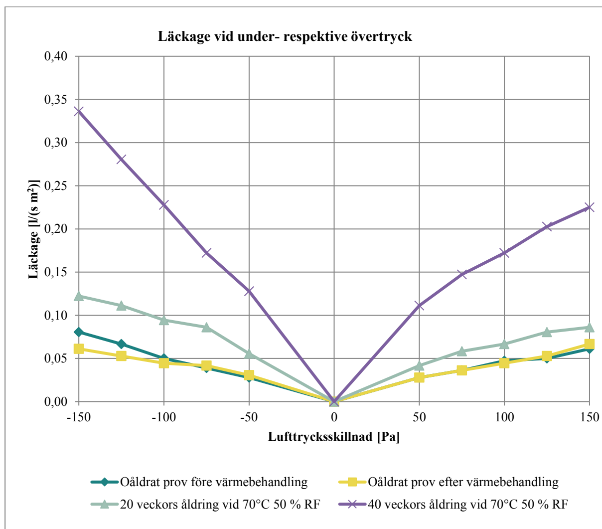
Diagram 18. Man ser att den inledande värmebehandlingen inte påverkar lufttätthetssystemet något nämnvärt. Långtidsåldringen påverkar dock systemet negativt vid 20 veckors åldring i ganska ringa grad för att sedan påverka i större grad vid 40 veckors åldring. Vid den, av leverantören av lufttätthetssystemet, valda åldringstemperaturen på 70°C kan genom att använda den så kallade Arrheniusekvationen göra ett antagande om att en användningstid om 25 år simulerats.
