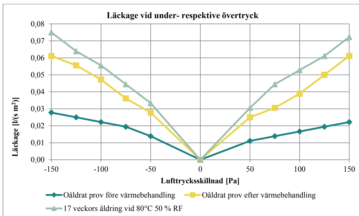
Diagram 27. Resultat från långtidsåldring av prefabricerad provvägg med polyuretanisolering.
