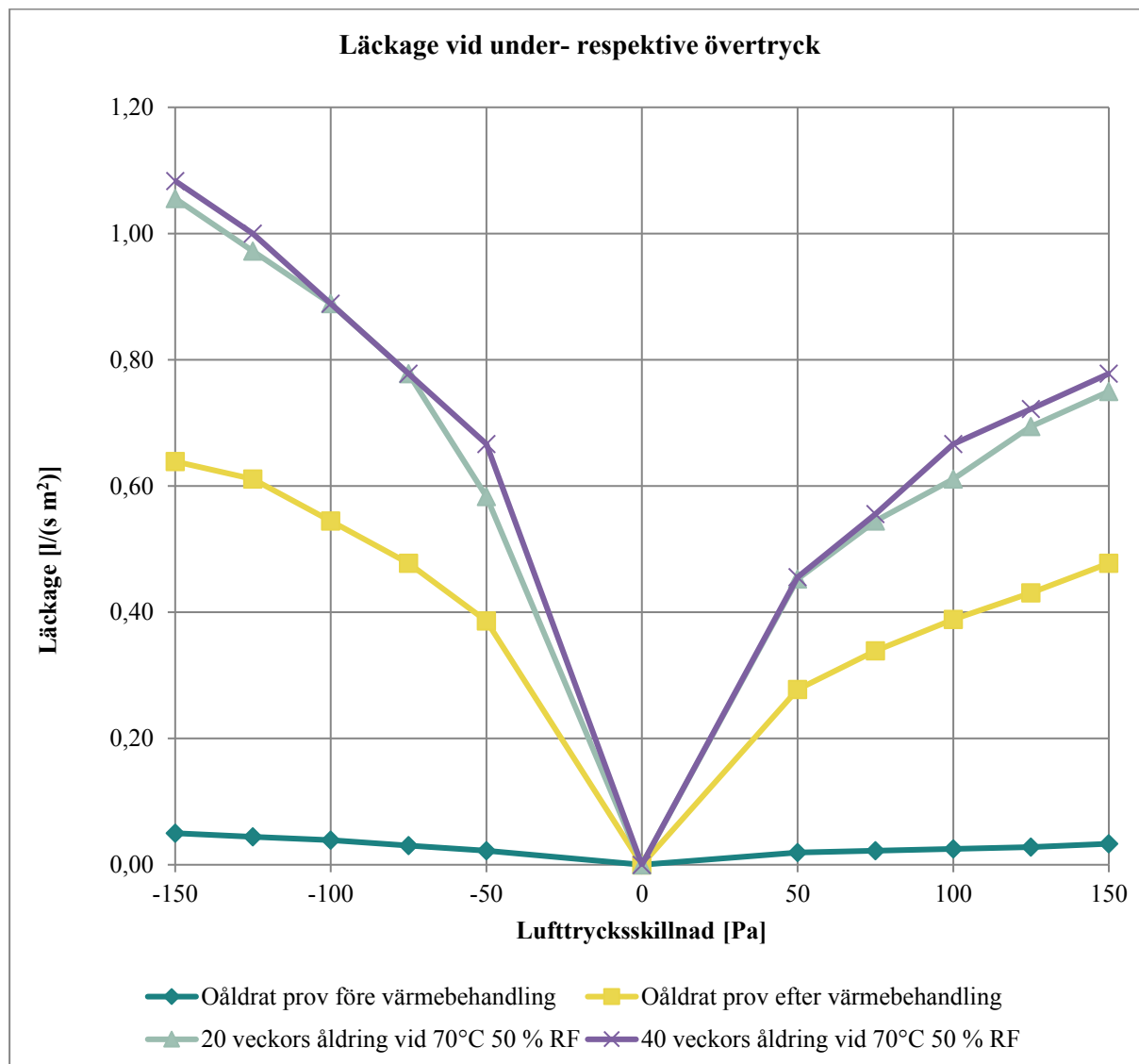
Diagram 11. Sammanställning av mätningar av luftläckaget då montage av lufttätessystemet har gjorts under ideala förhållanden och därefter långtidsåldring under 40 veckor vid 80°C 50 % RF.
