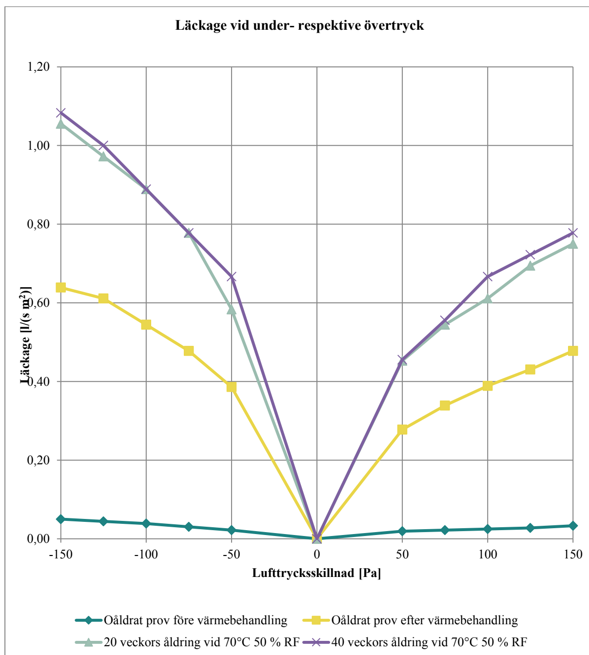
Diagram 26. Man ser att den inledande värmebehandlingen påverkar lufttätthetssystemet ganska kraftigt. Långtidsåldringen påverkar också systemet negativt, vi ser dock ingen större förändring mellan 20 veckors åldring och 40 veckors åldring.
