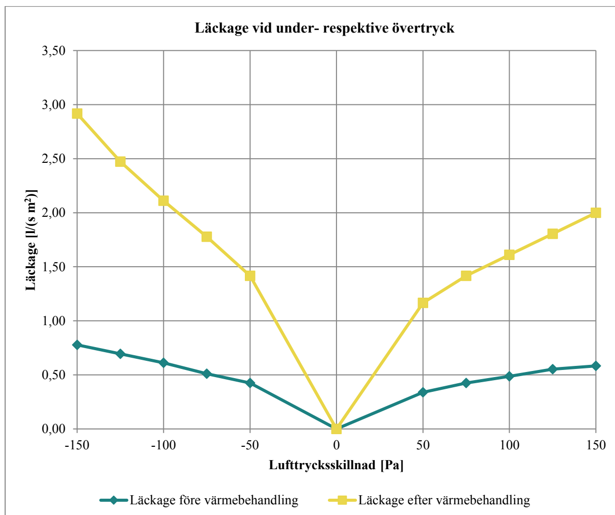
Diagram 24. Lufttätethetssystem 3 visar en relativt stor förändring av lufttäteten efter montage i klimat, denna förändring syns dock först efter värmebehandling.
