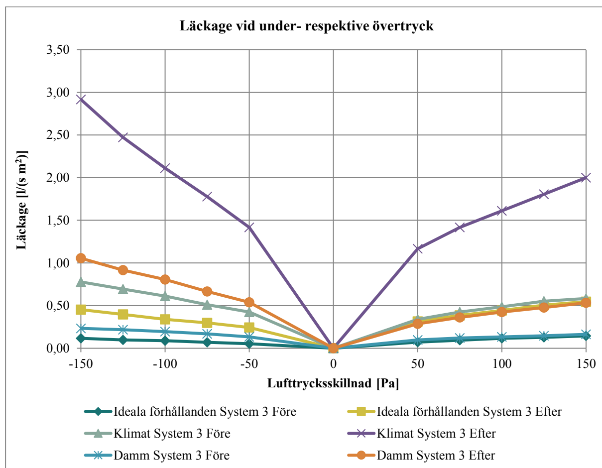
Diagram 10. Sammanställning av mätningar av luftläckaget då montage av lufttätetsystemet har gjorts under olika förhållanden.
