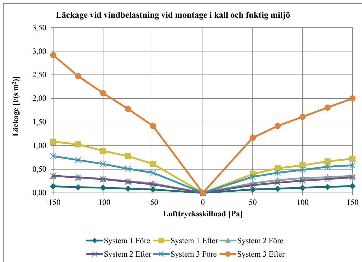
Diagram 2. Alla de undersökta lufttätethetsystemen visar på förändringar i lufttäteten efter värmebehandlingen då montaget hade skett i kall och fuktig miljö. Variationen mellan de olika systemen var dock ganska stor.
