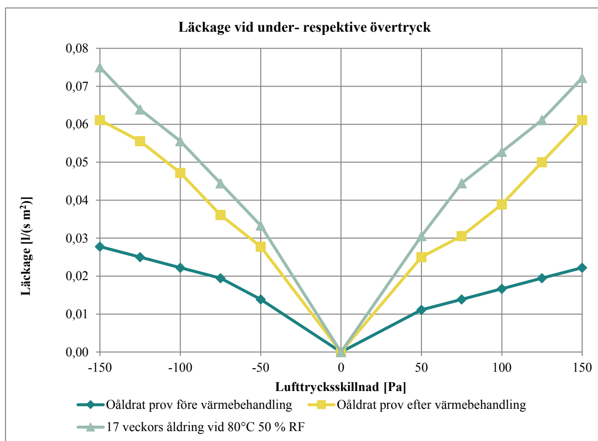
Diagram 12. Resultat från långtidsåldring av prefabricerad provvägg med polyuretanisolering.
