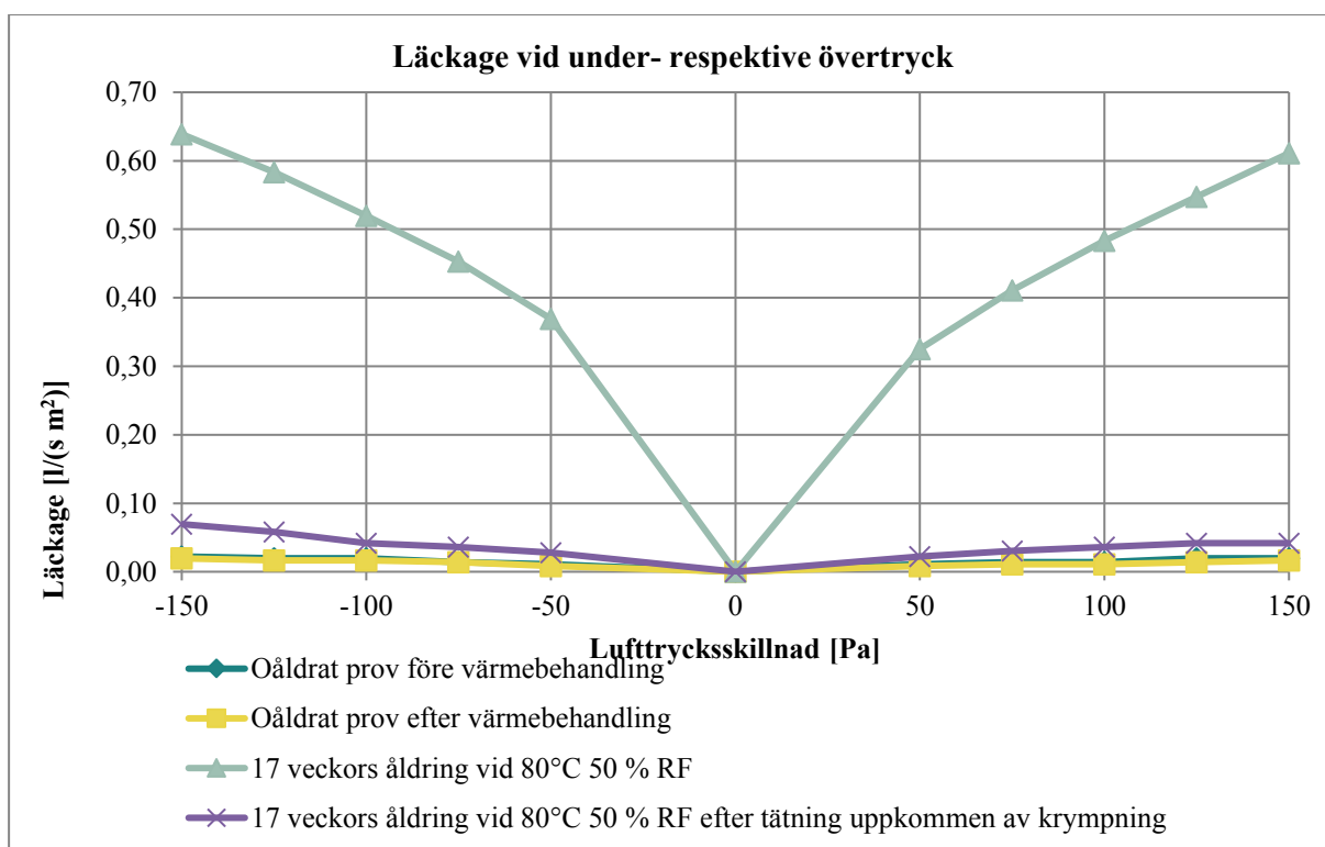
Diagram 28. Resultat från långtidsåldring av in-situ tillverkad provvägg med polyuretanisolering.
