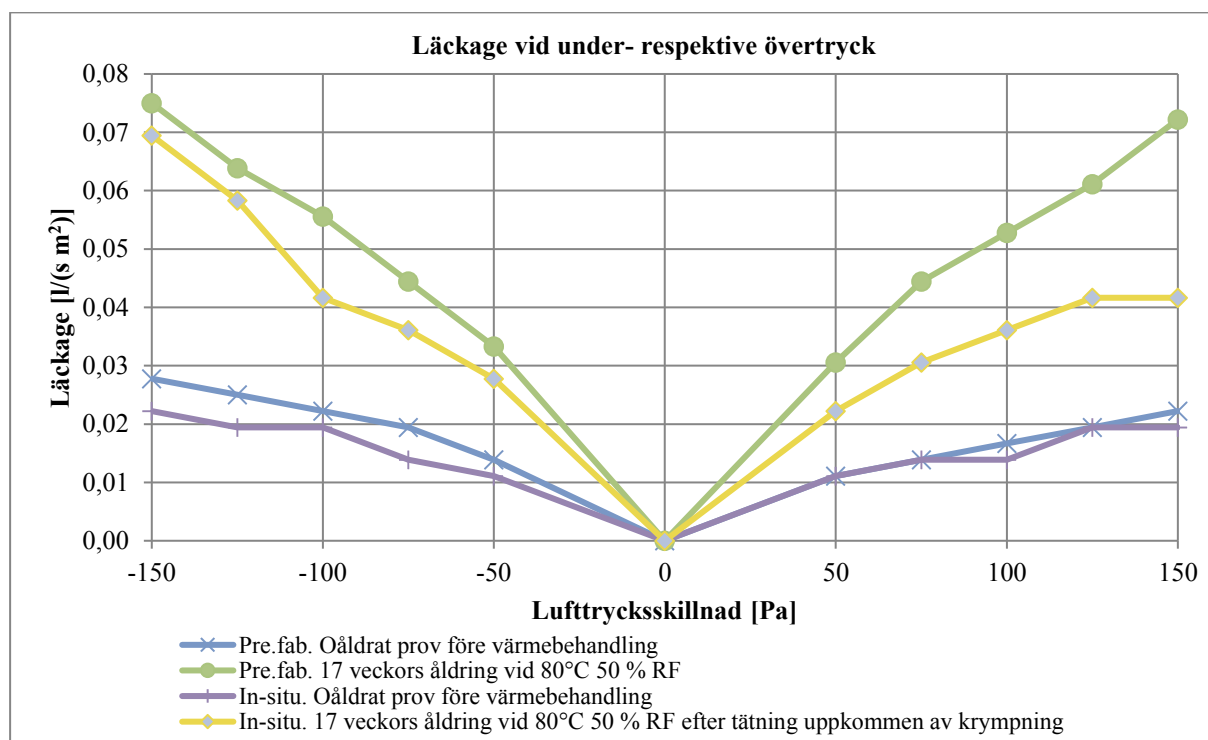
Diagram 5. Diagrammet visar att både prefabricerad och in-situ applicerad polyuretanisolerings är mycket lufttät både initialt och efter långtidsåldring under 17 veckor vid 80°C 50 % RF.
