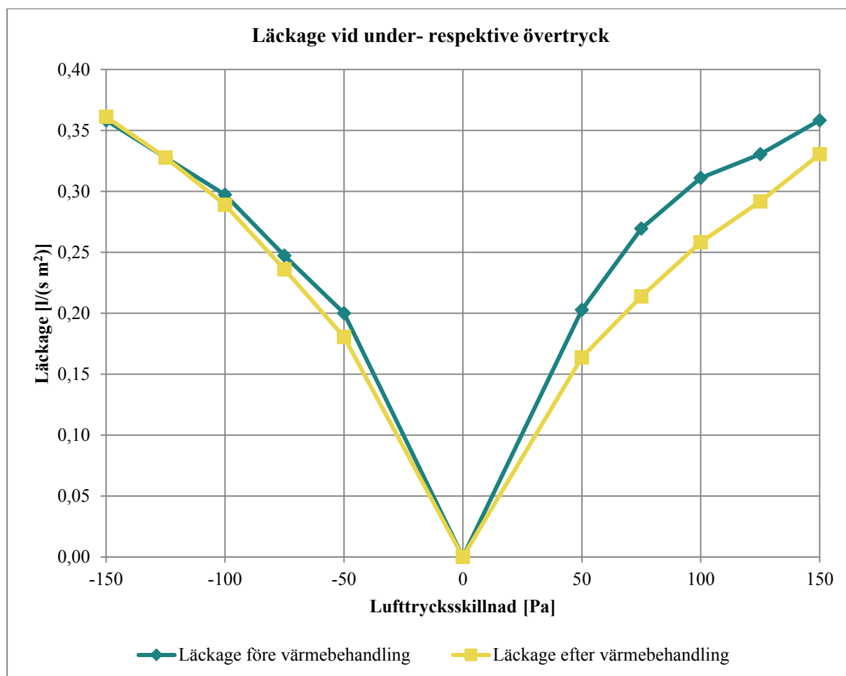
Diagram 20. Lufttätethetssystem 2 visar på förändring vid montage i kallt och fuktigt klimat. Värmebehandlingen påverkade inte lufttätethetssystem 2 i någon negativ riktning. Förändringen är mindre än hos lufttätethetssystem 1 och 3.
