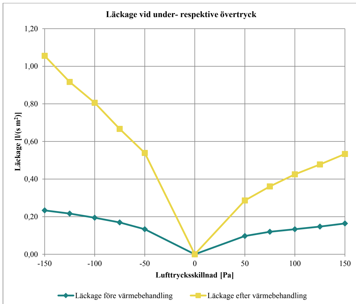
Diagram 25. Lufttätessystem 3 visar förändring av lufttäteten efter montage i dammig miljö, denna förändring syns dock först efter värmebehandling.
