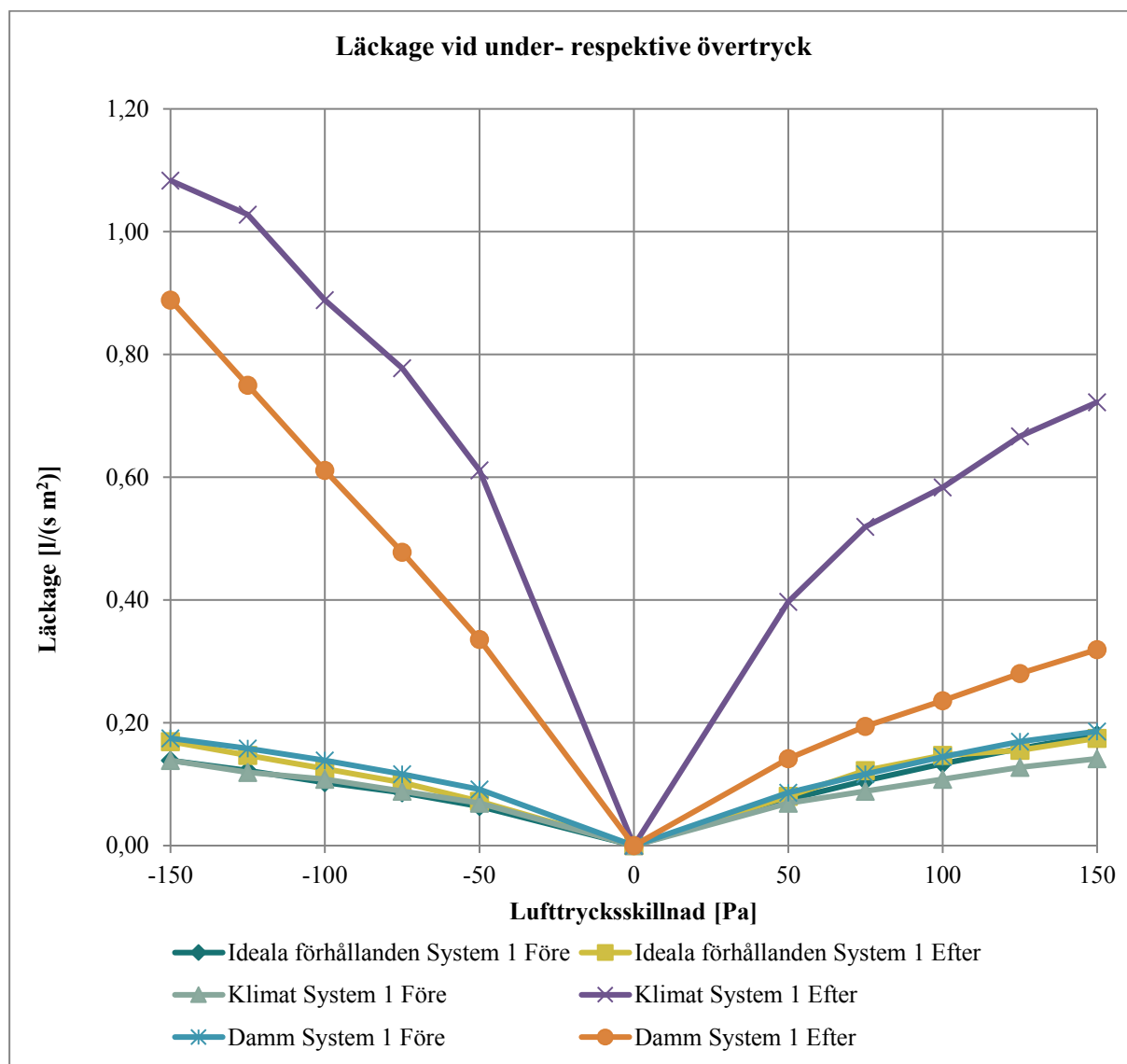
Diagram 6. Sammanställning av mätningar av luftläckaget då montage av lufttätetsystemet har gjorts under olika förhållanden.
