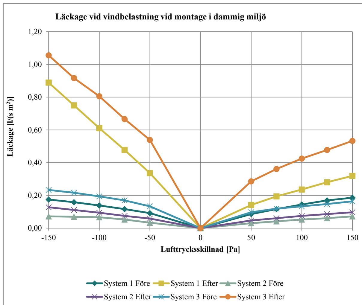
Diagram 3. Vid montage i dammig miljö uppvisar lufttätethetssystem 1 och 3 en relativt stor förändring, denna förändring syns även här dock först efter värmebehandling.
