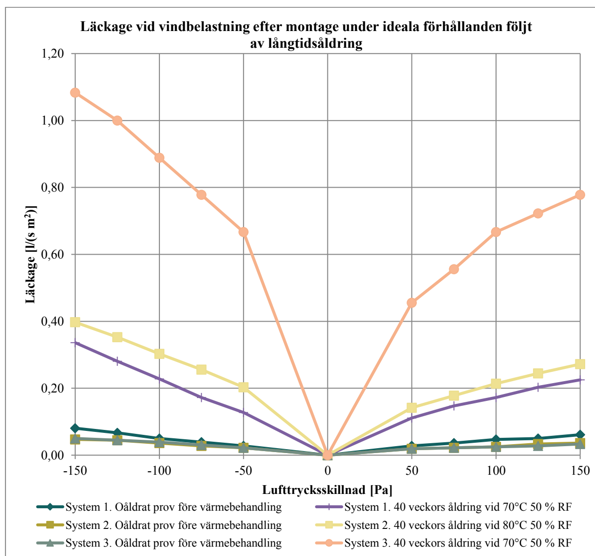
Diagram 4. Diagrammet visar på stor spridning i läckage mellan olika lufttätethetsystem. Notera att kurvorna för de oåldrade lufttätethetsystemen 2 och 3 ligger i varandra.
