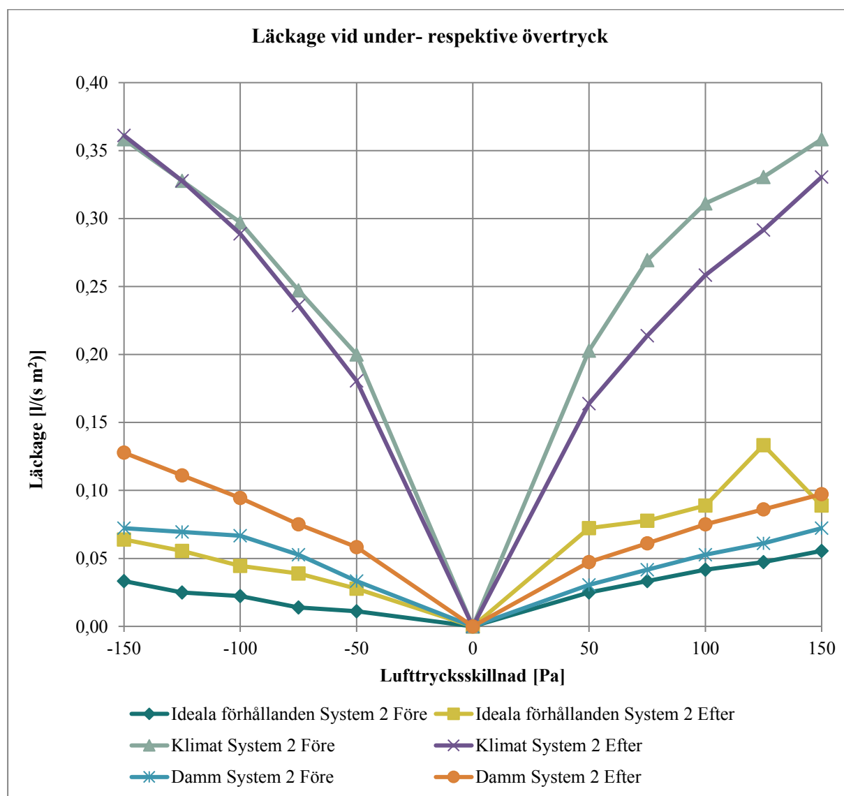
Diagram 8. Sammanställning av mätningar av luftläckaget då montage av lufttätetsystemet har gjorts under olika förhållanden.
